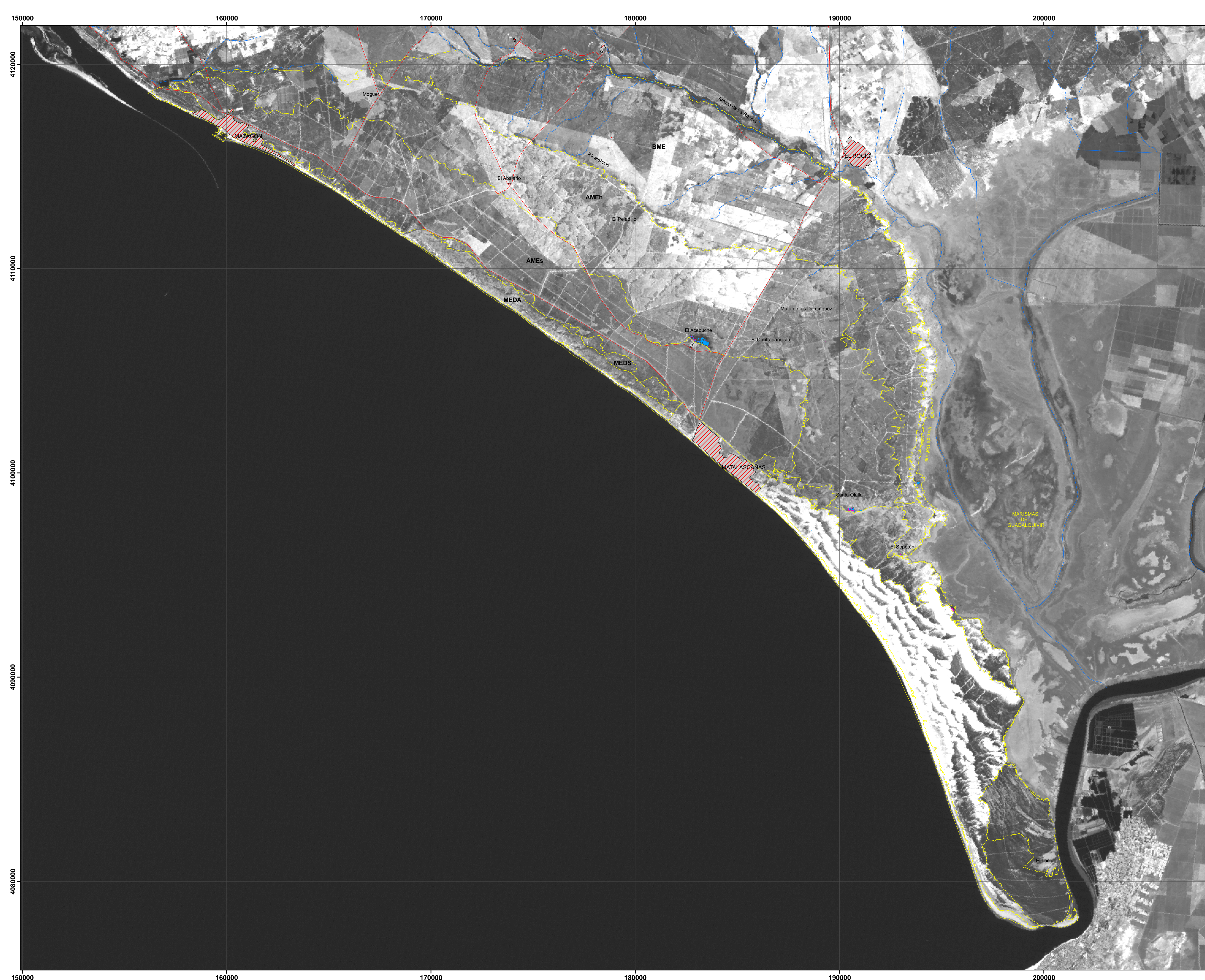
Cartografía de lámina de agua y superficies encharcadas. Septiembre 1994. Landsat TM
